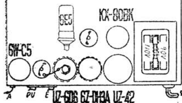
真空管配図
