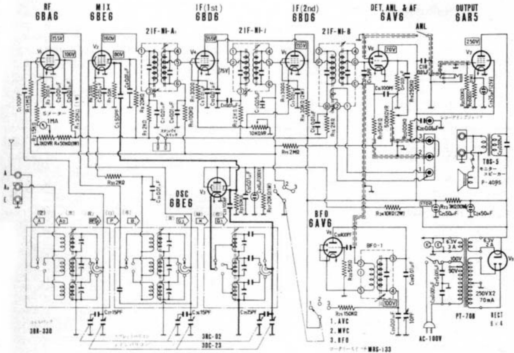
CRV-1 回路図
