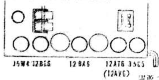
真空管配置図
