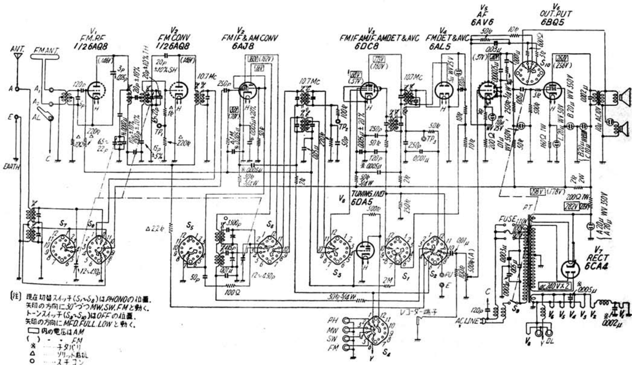
ナショナル EA-765 型受信機の回路図
