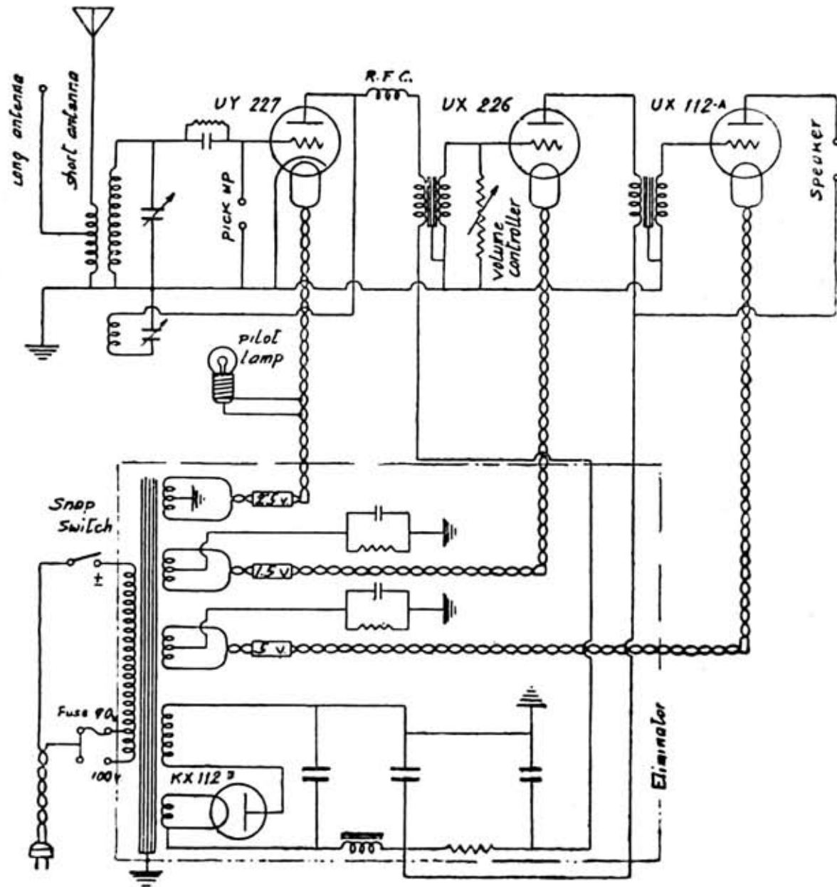
ナショナル四球交流受信機配線圖 音量調節式
