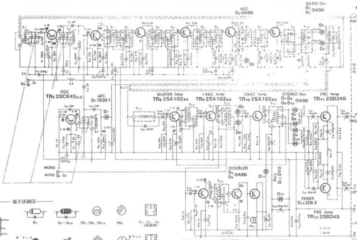
「ナショナル」CJ-951 回路図
