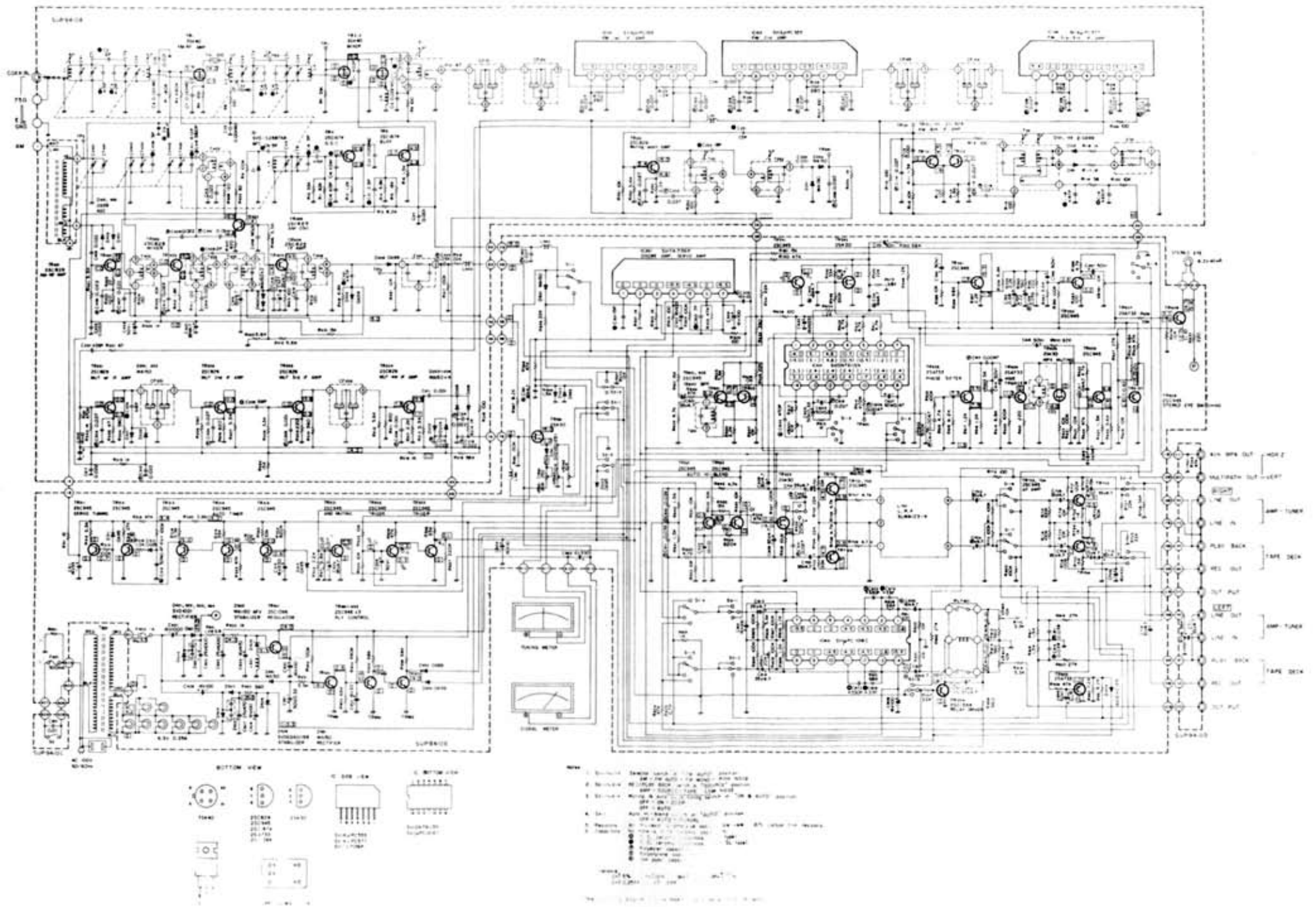
FM ステレオチューナST-8600の回路図
