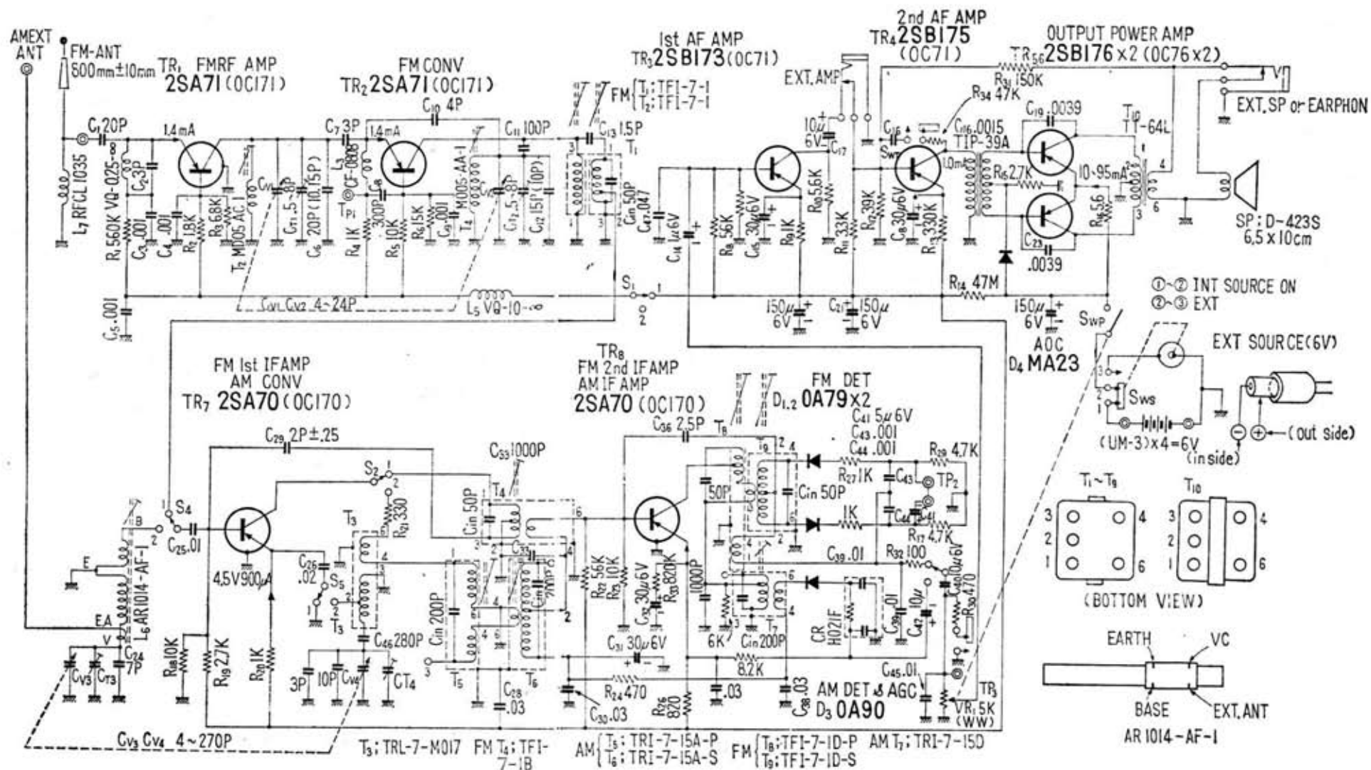
ナショナル T-81 FM/AM 8石トランジスタラジオの回路
