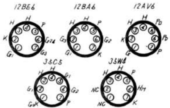
真空管挿接図(左視)
