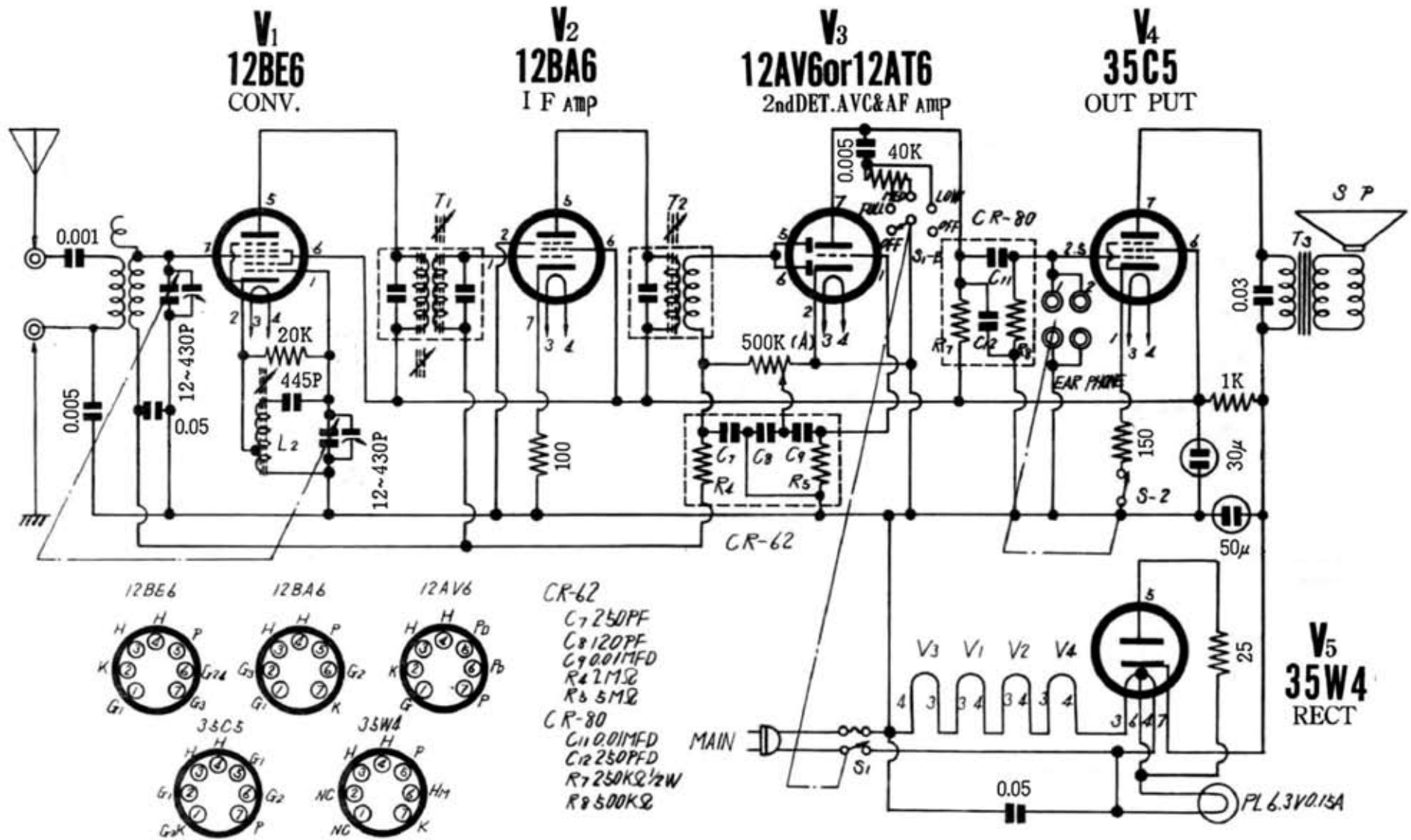
真空管挿接図(左視)
