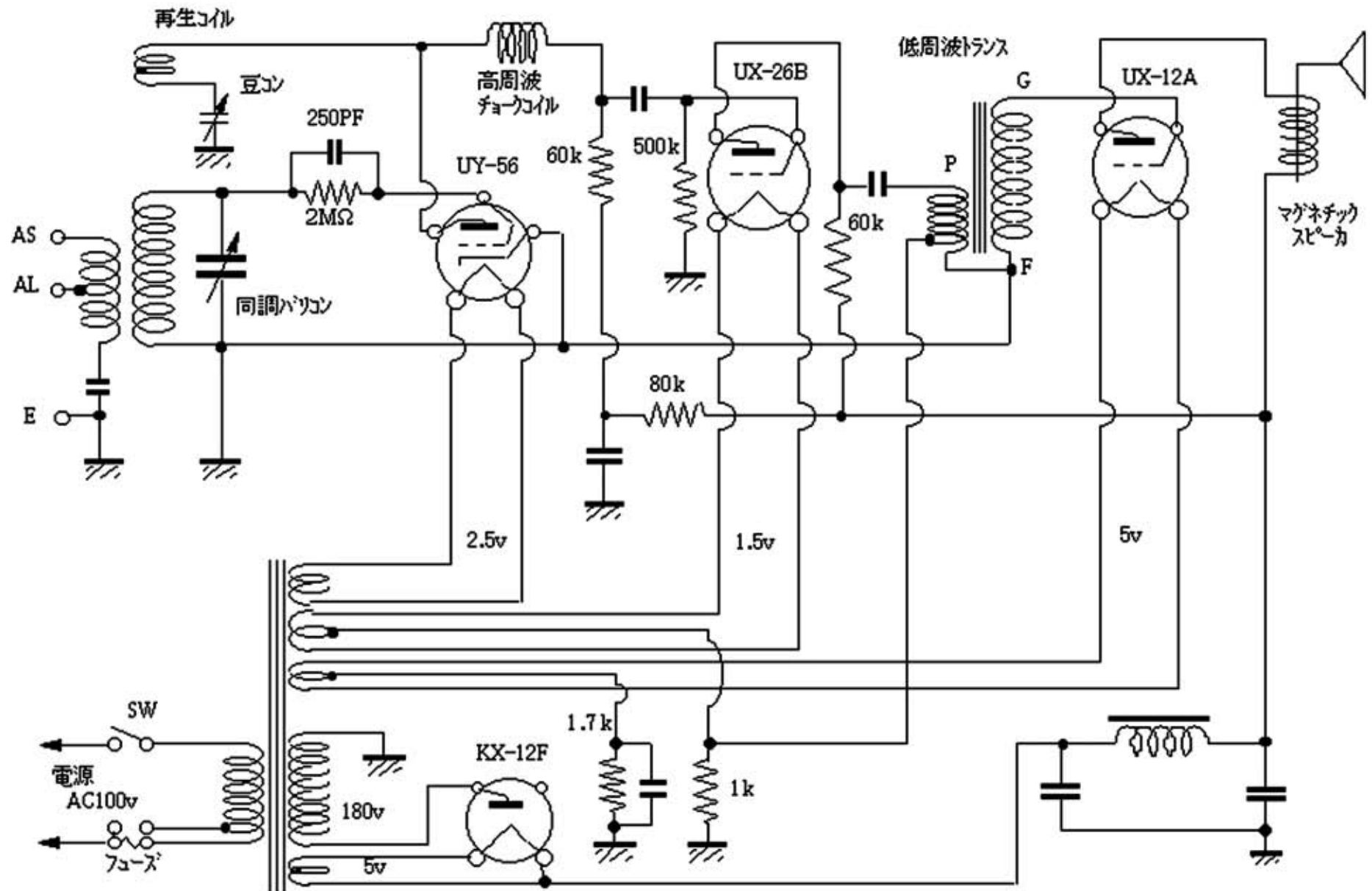
Z-20型 ナショナル国民受信機 (再生式 4球) 回路図
