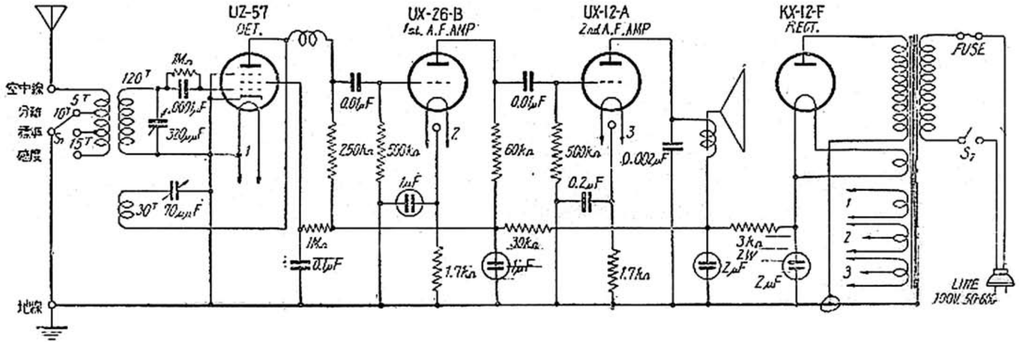
第 1 圖 (國策 I 號型受信機の全回路結線圖。)
