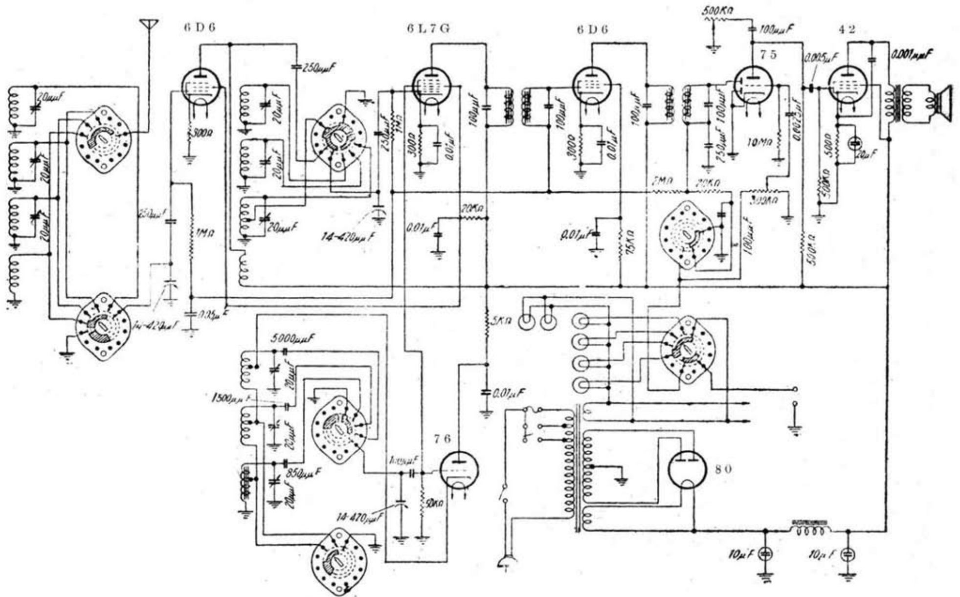
7A-1型7球式全波受信機配線圖
