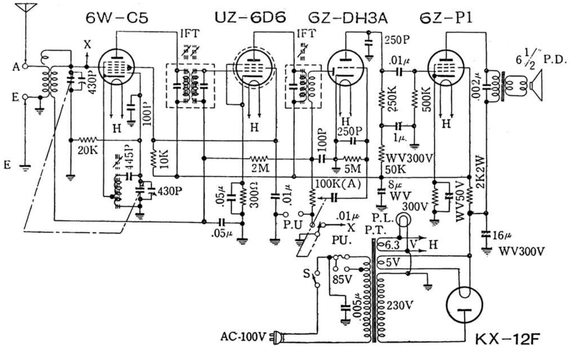
図解ラジオ文庫「4・5球スーパーの組立と調整」
