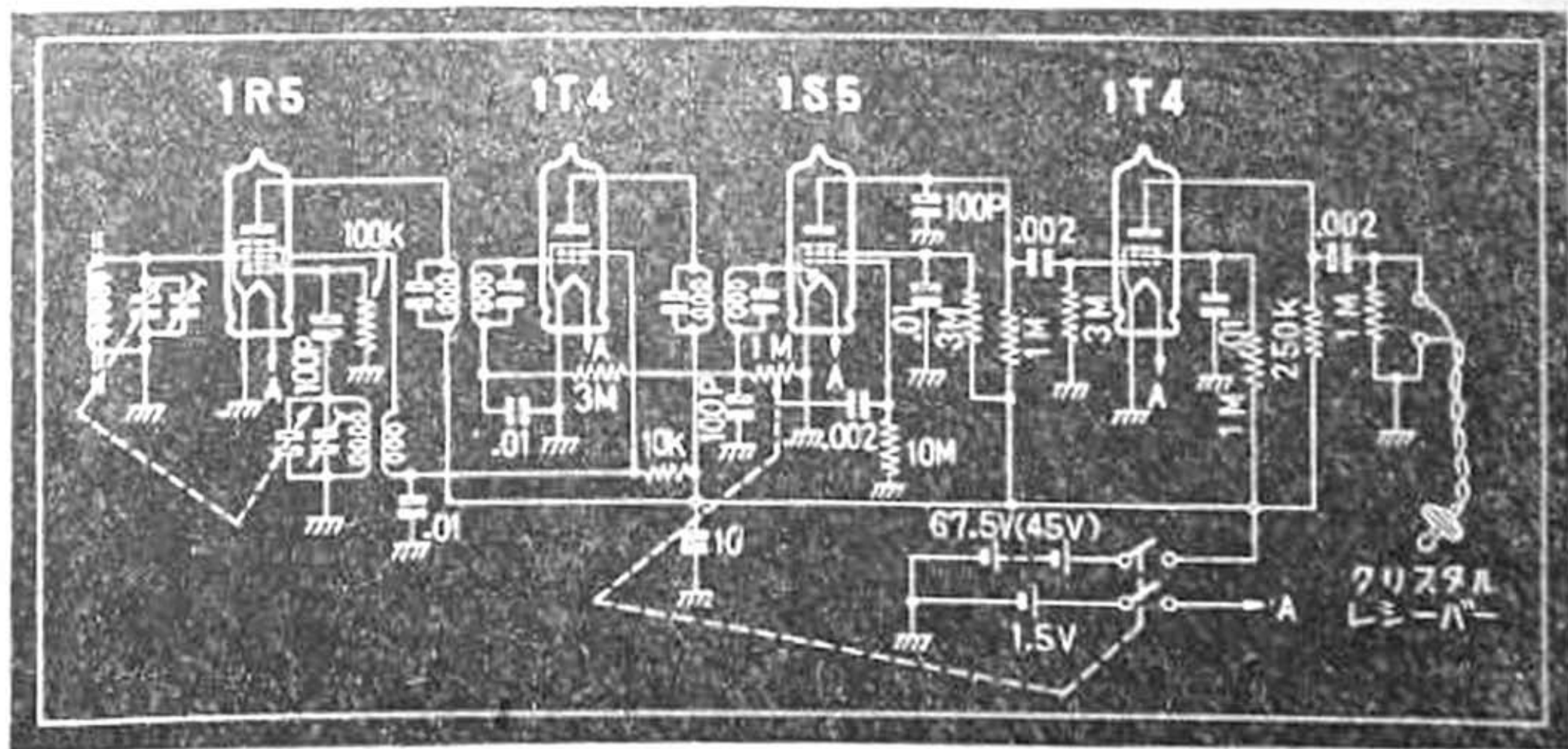
RN-2, AF-2段, 4球スーパー・ポケット・ラジオ
