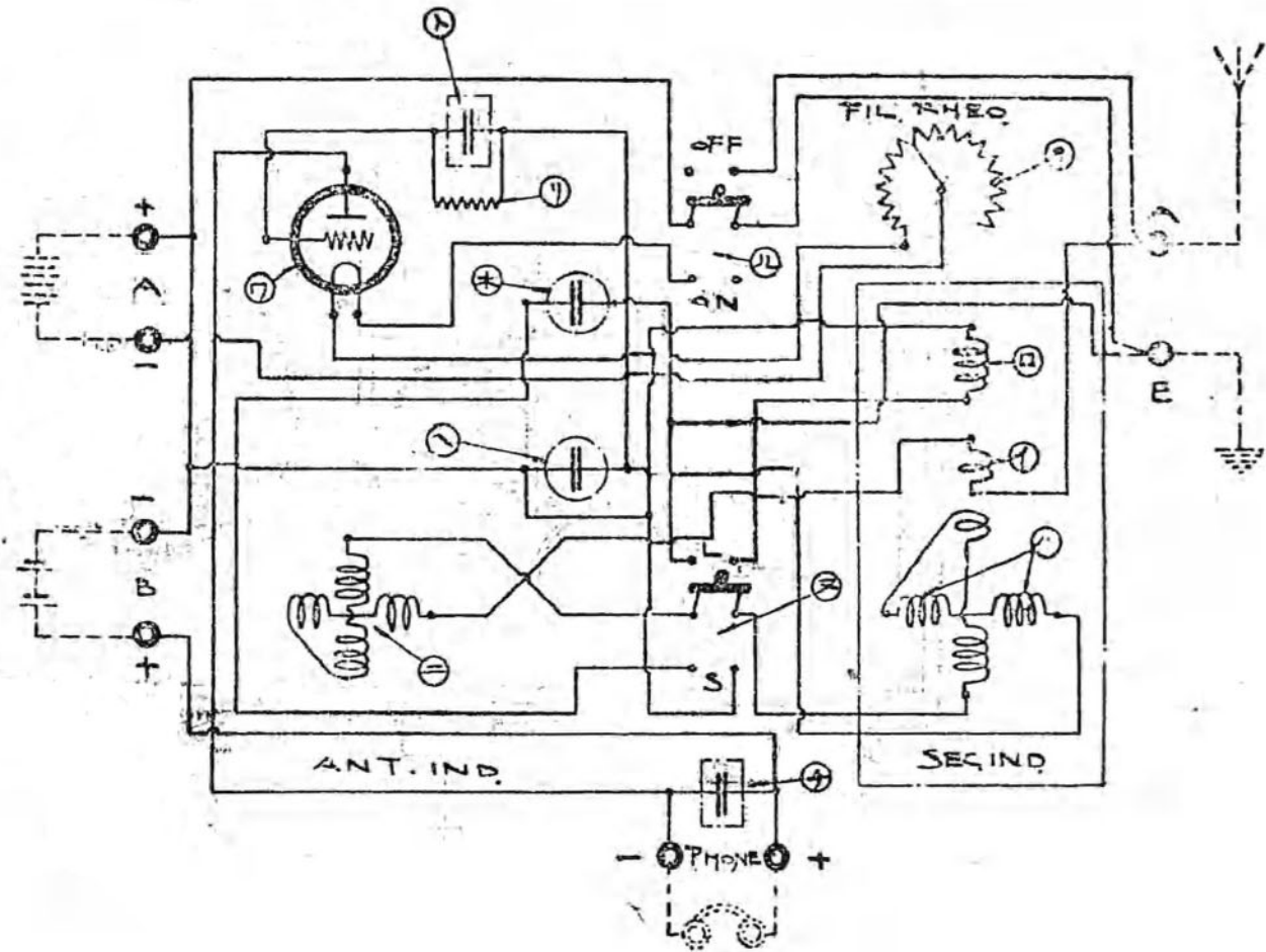
沖式一號受信機
