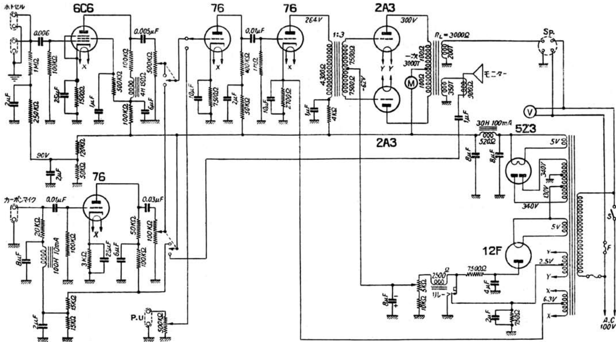
東京音響製 15 W トーキー、マイク、フォノ用擴聲機
