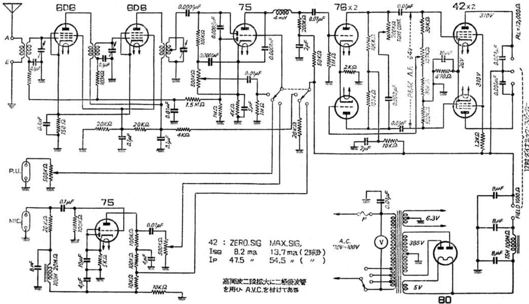
東京音響製 8.5 W ポータブル 擴聲機
