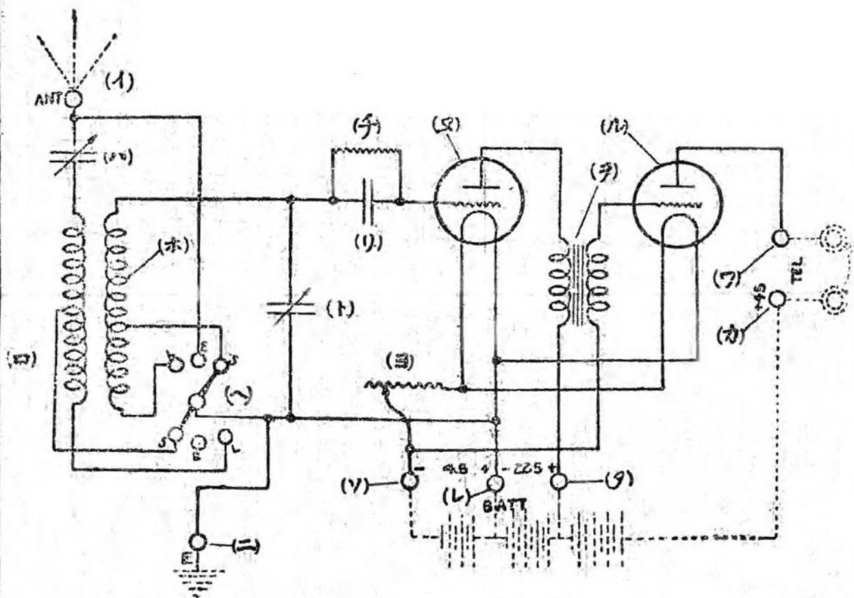
「サイモフオーン」A-2型受信機
