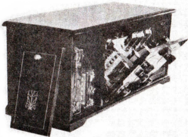
サイモホンC型の内部
