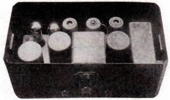
オリオン 300 號受信機の内部
