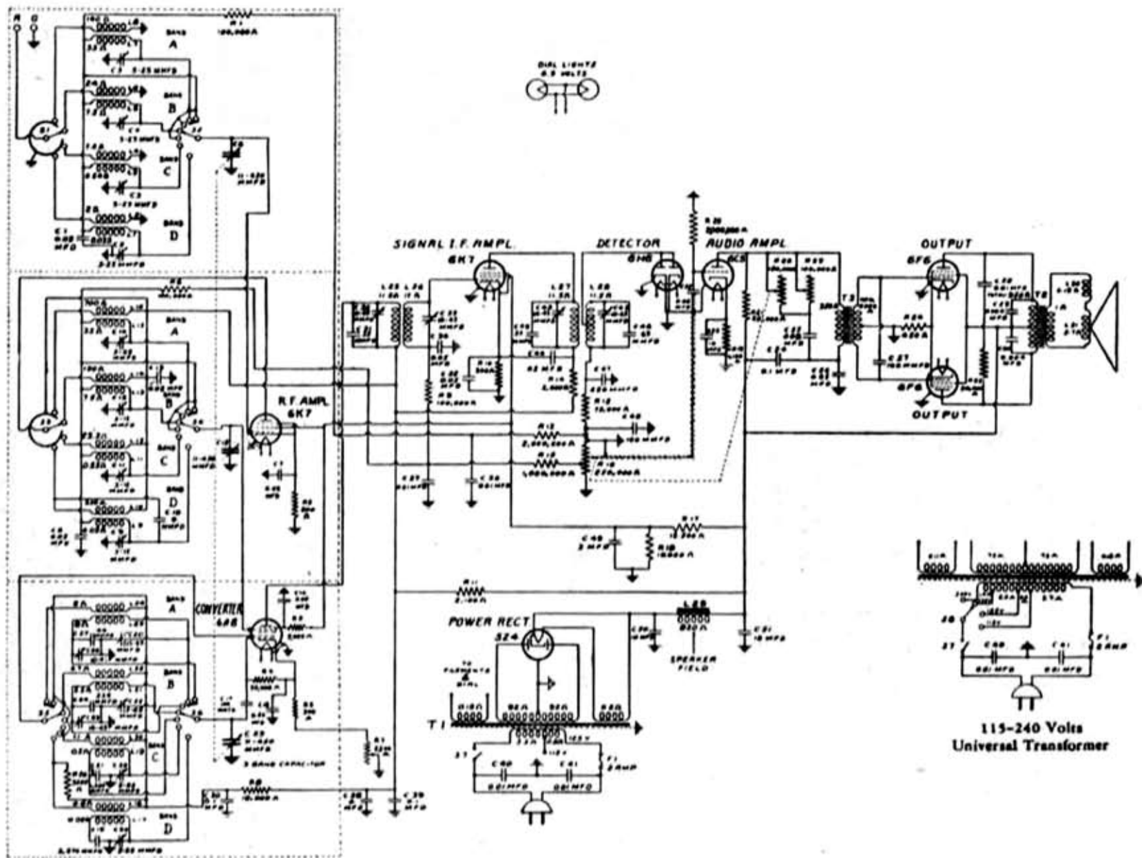
A-82型受信機の配線図
