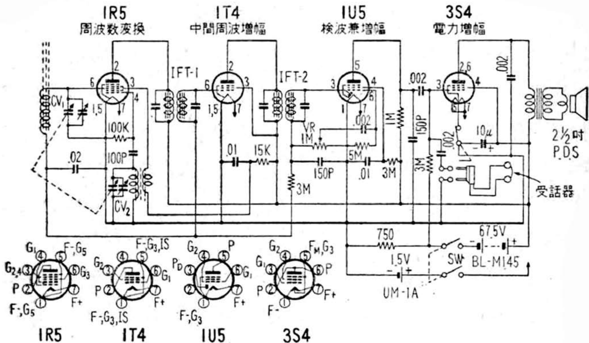
オータ OPR-120 型 4球ポータブル・ラジオ配線図
