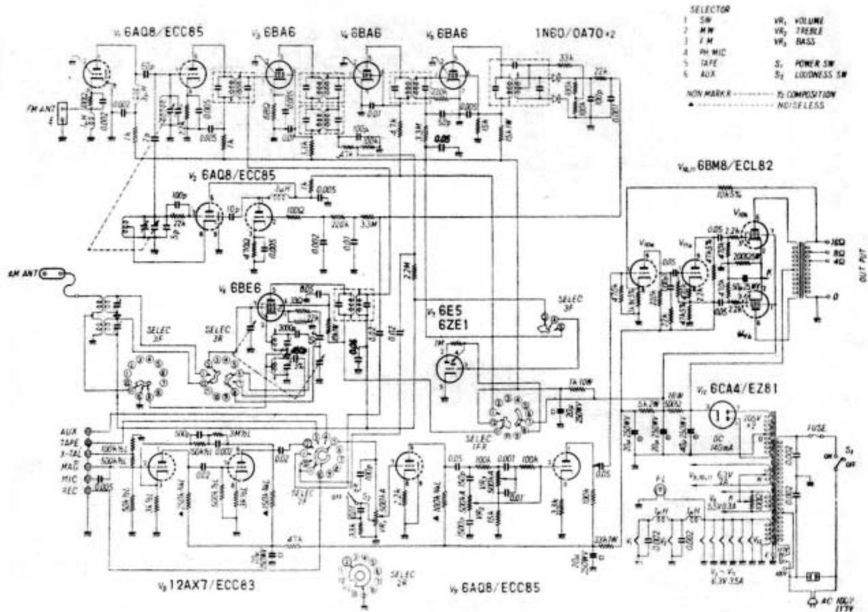
FM-B302 の回路図
