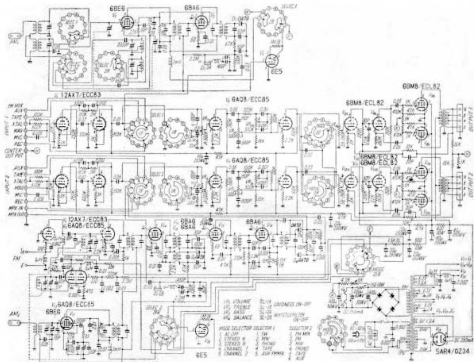
SM-B201 の回路
