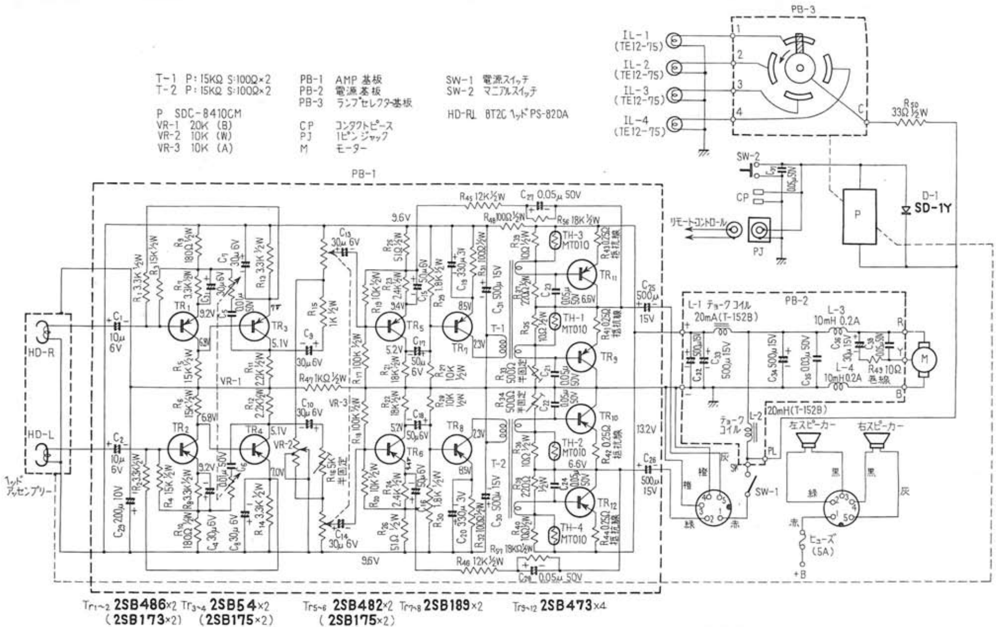
「パイオニア」TP-80 回路図
