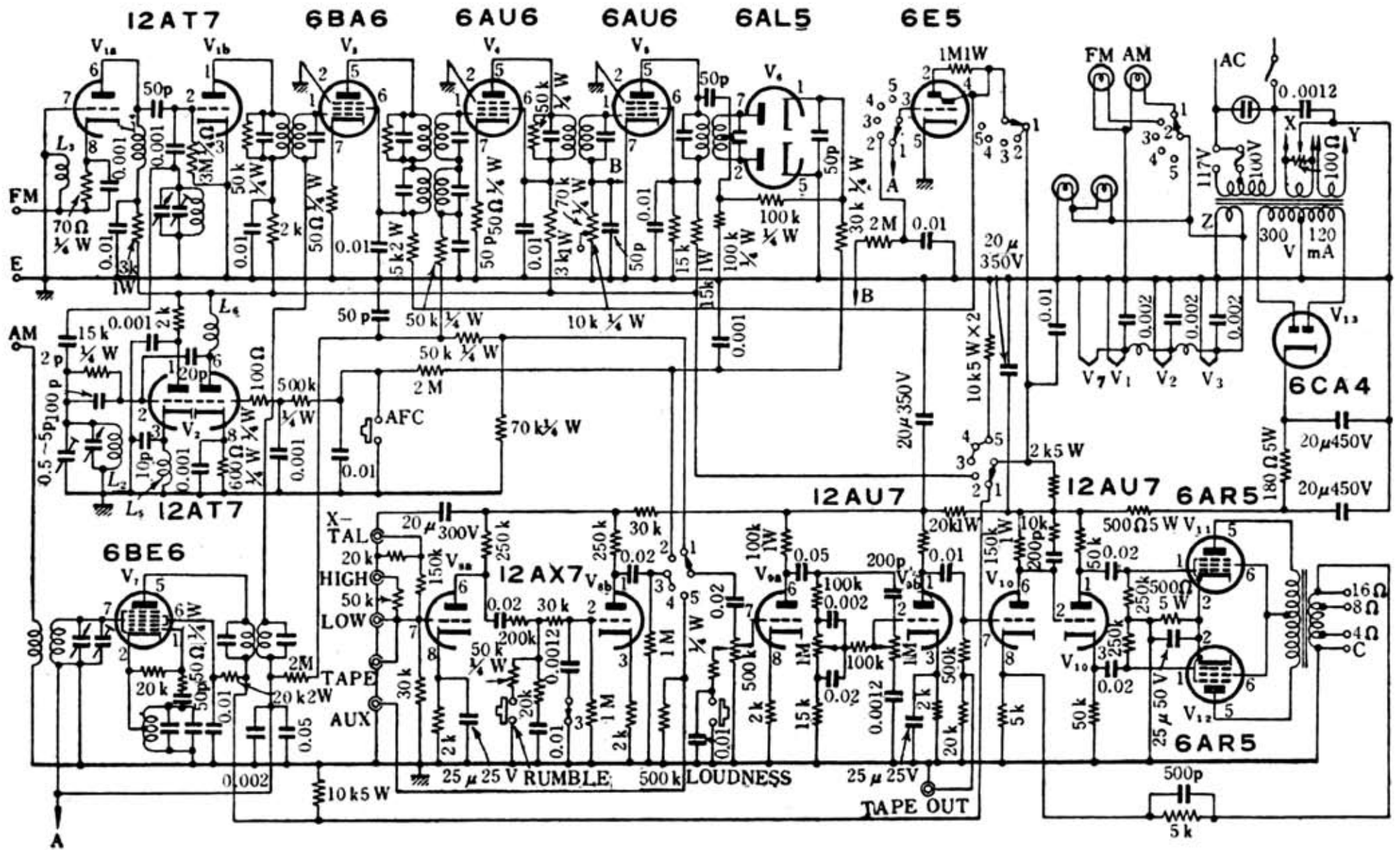
山水電機 PM-800 型 AM-FM 受信機
