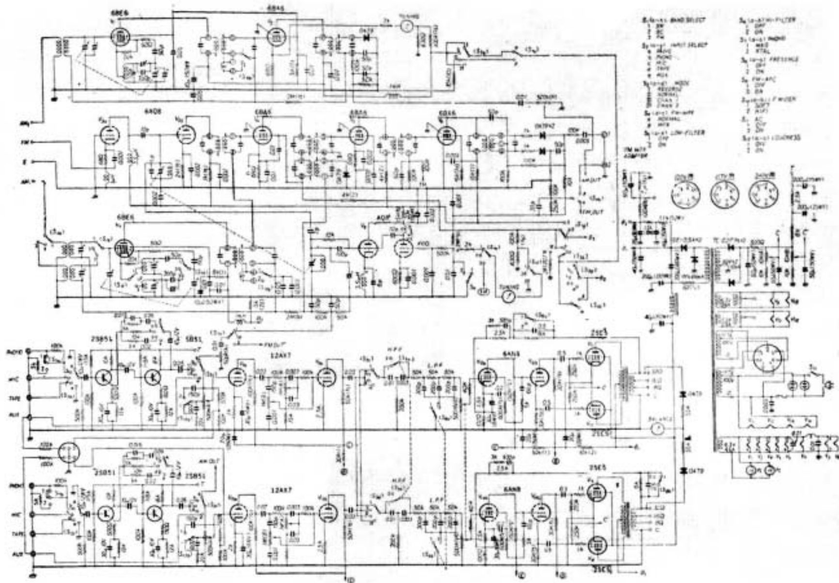
SM-80 の回路
