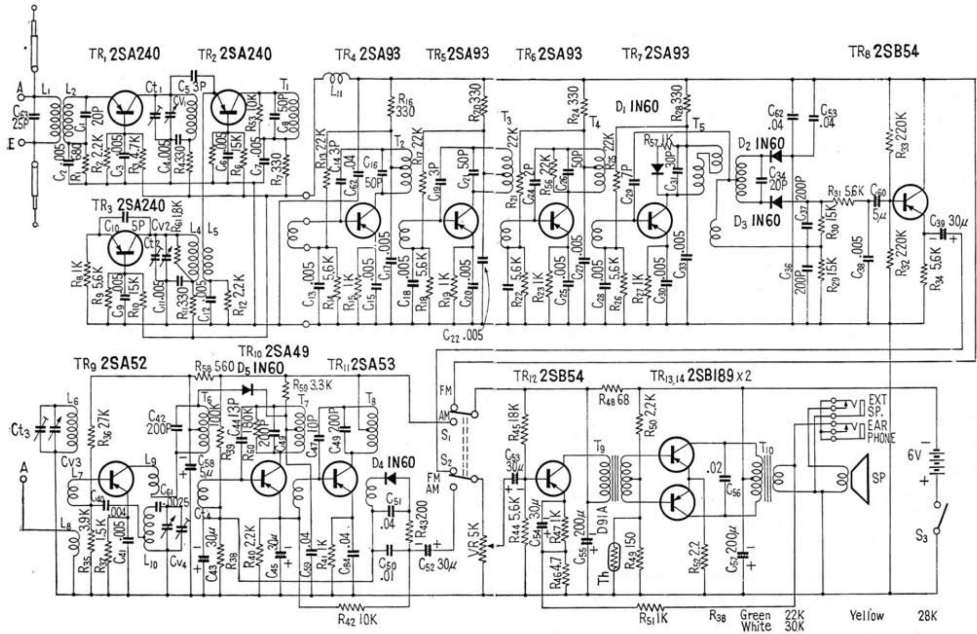
三洋 AFT-1 A 形 FM/AM 14, トランジスタラジオの回路
