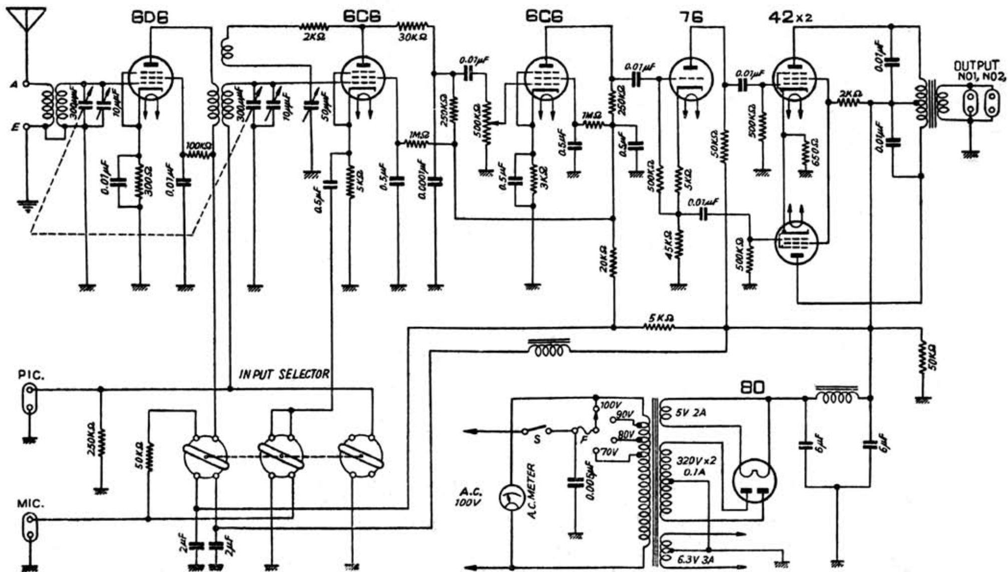
早川電機工業製 [シャープ, RA-8型] 携帯用増幅機
