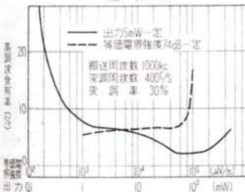
歪特性
