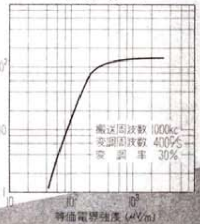
出力特性
