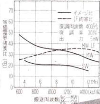
映像・中間周波妨害比特性
