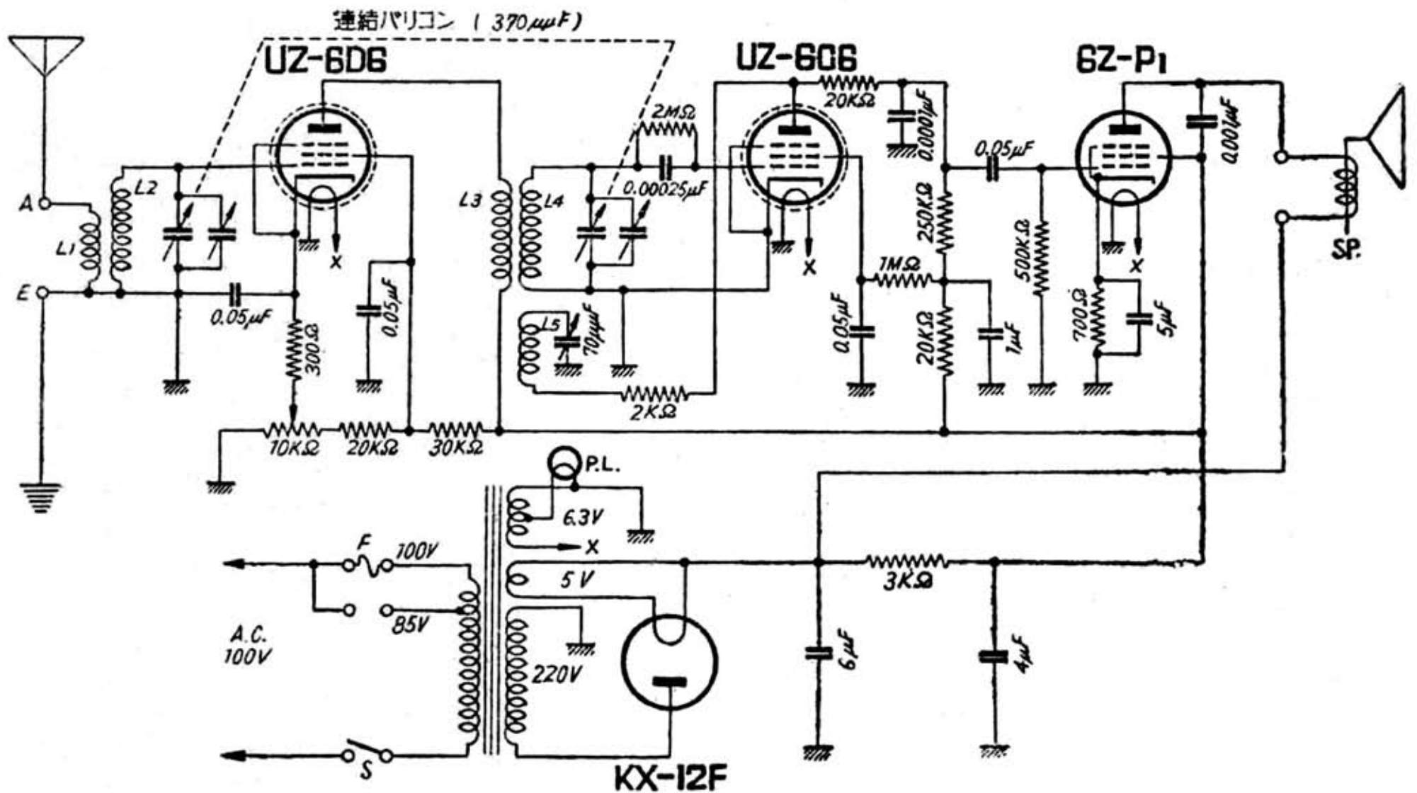
早川電機工業製 [シャープ] 国民2号A型受信機
