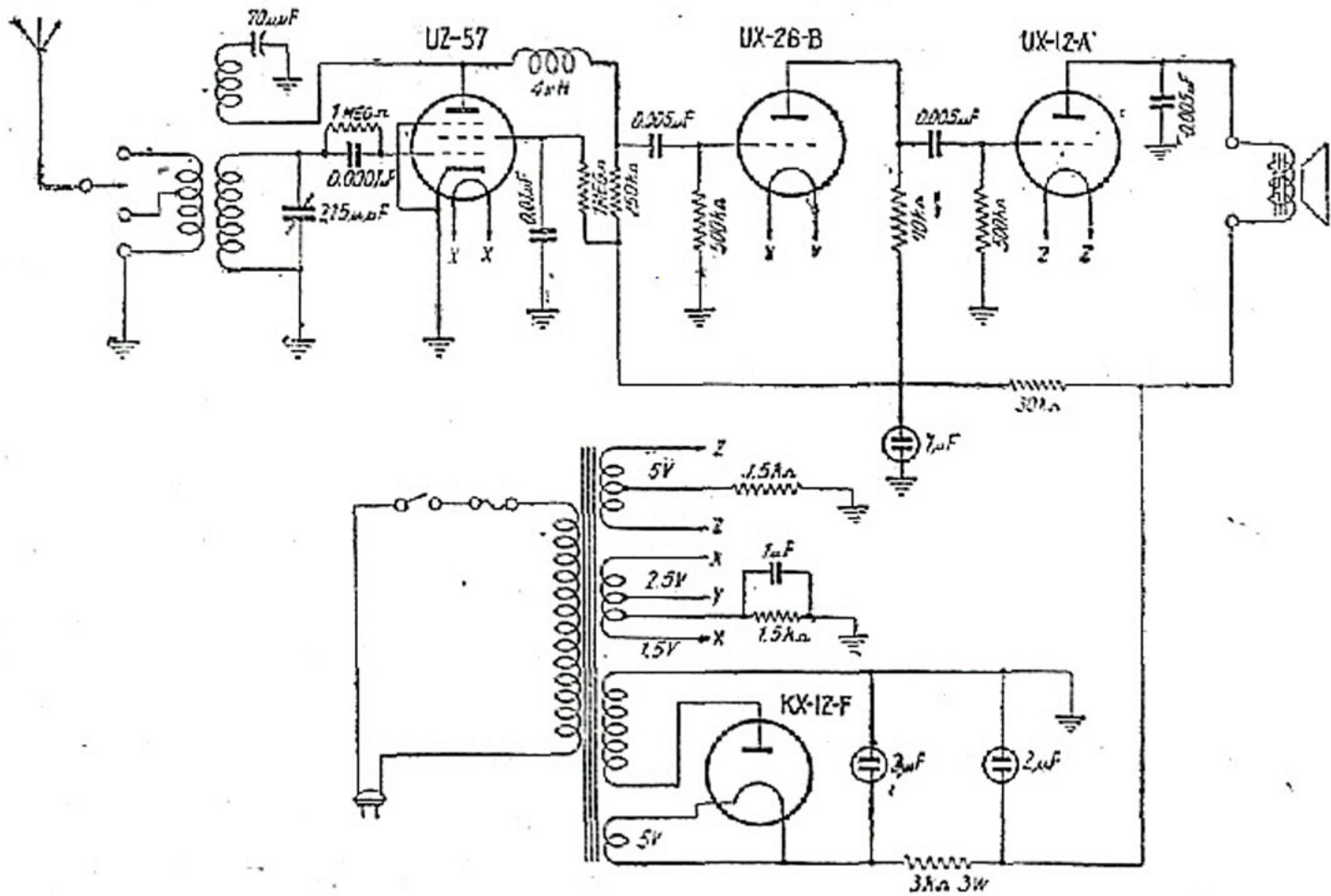
第 1 圖 [解剖したシャープ「國策-1 號型」受信機の回路結線圖.]
