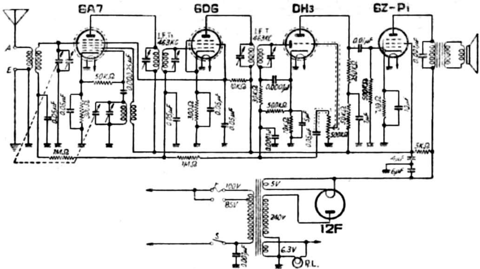
早川電機製 シャープ 5-R 型 5 球式スーパーヘテロダイン受信機
