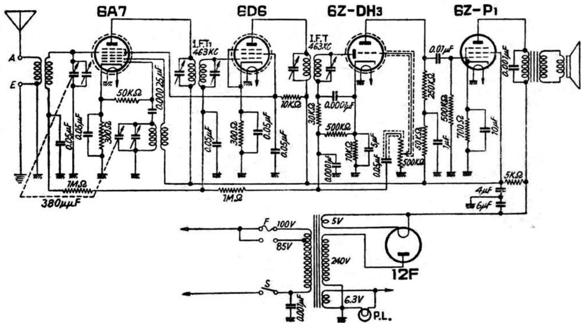
早川電機製 [シャープ5-R型] 5球スーパーヘテロダイン受信機
