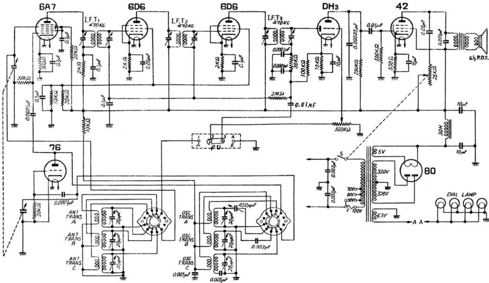
早川電機製 [シャープ7-S型] 7球オールウェーブ受信機
