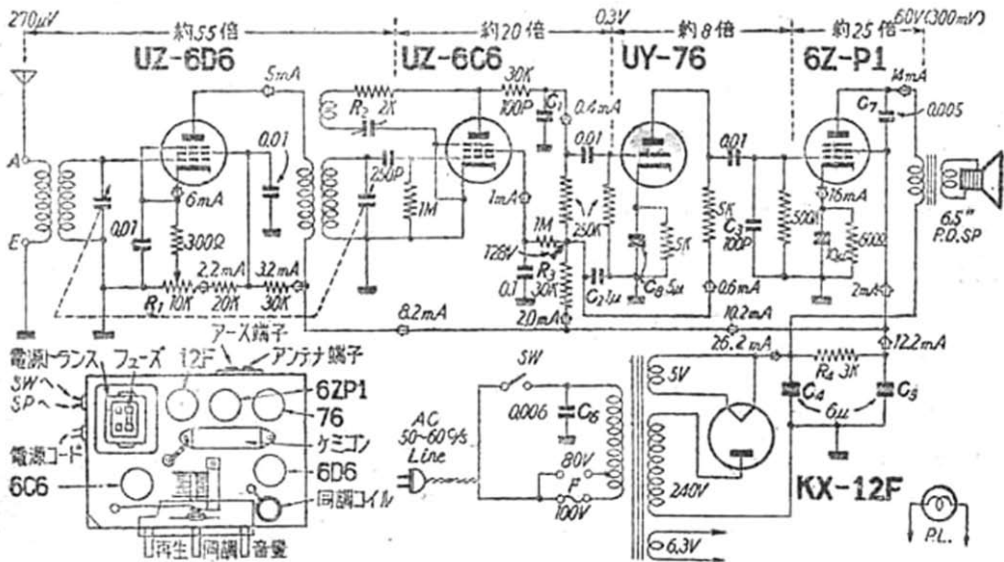
早川電機製国民型受信機〔5H-16型〕回路図
