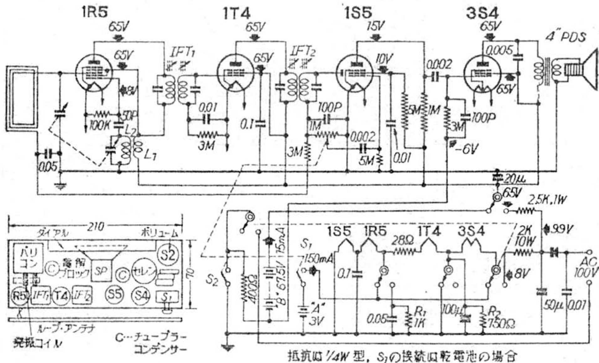
シルバー 50W 4 型受信機回路図
