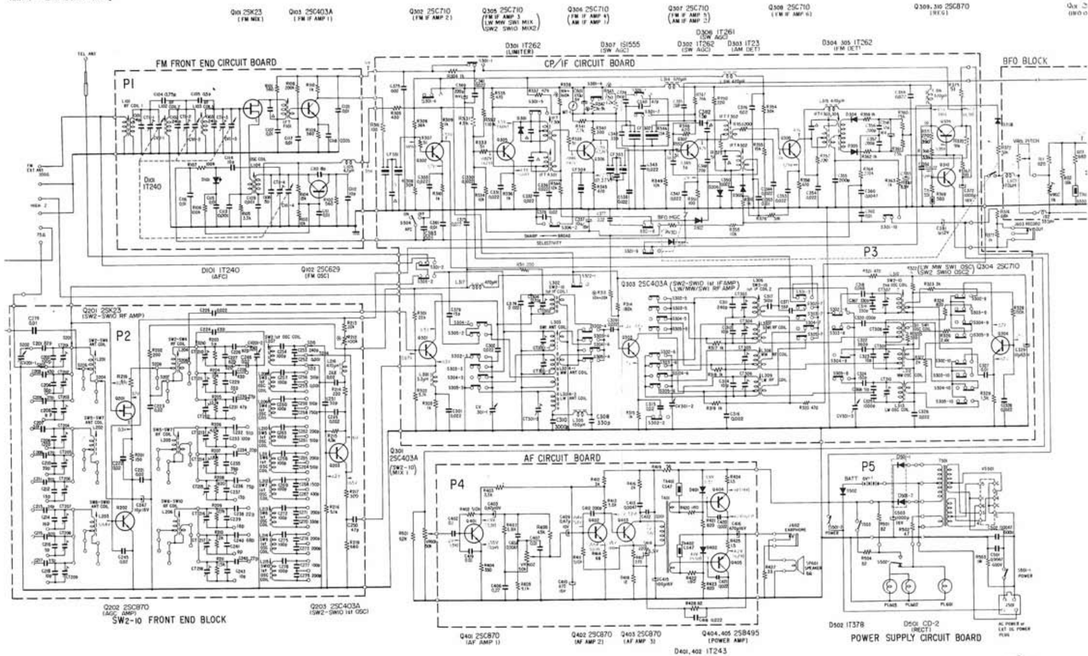
回路图·電圧電流分布图
