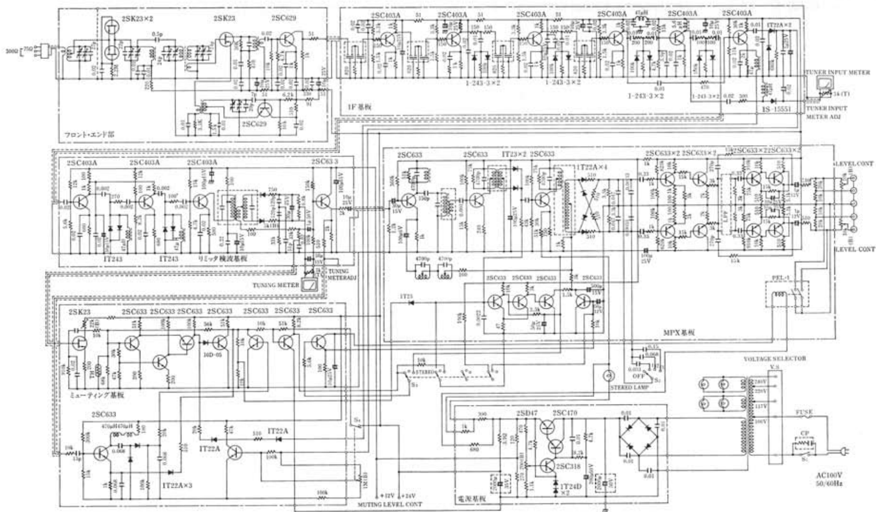
高級FMステレオ・チューナー (ソニーST-5000F 1969年)
