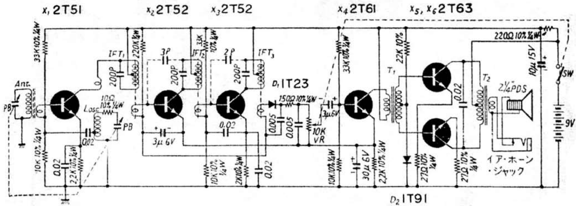
ソニー・トランジスタ・ラジオ・TR-63 の全回路図
