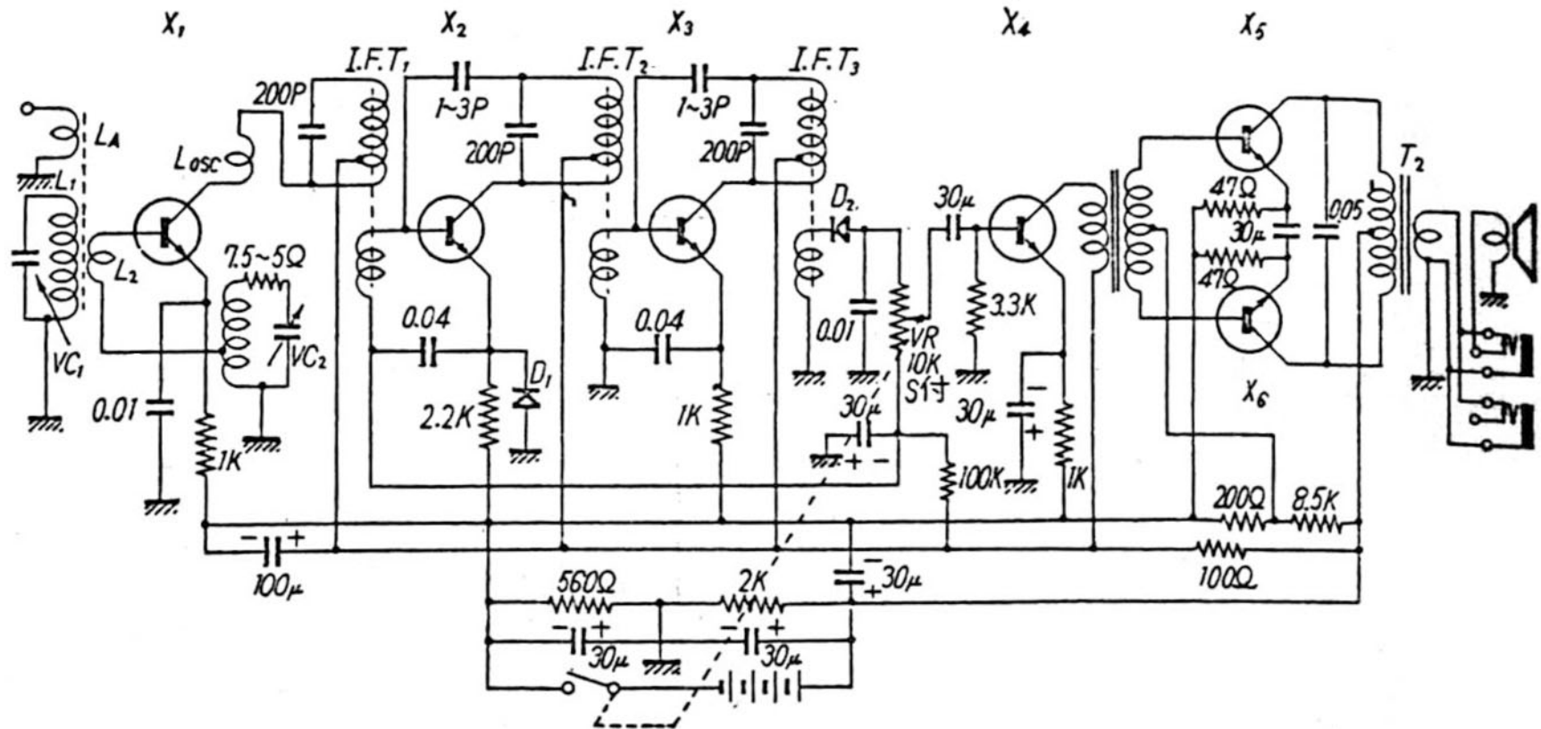
〈東通工 TR-6 型 6 石式〉
