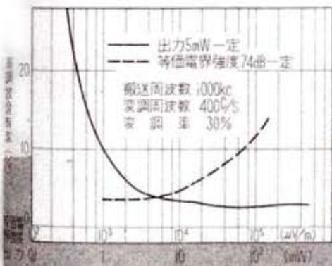
歪特性
