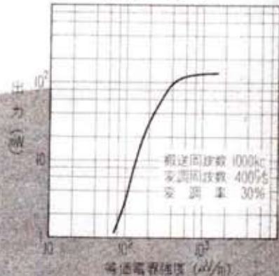
出力特性
