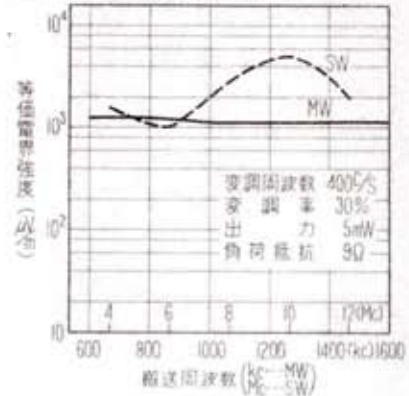
出力特性
