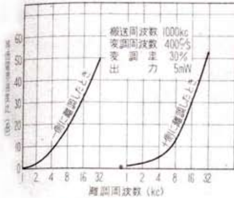
自動利得調節特性
