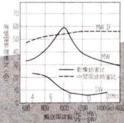
映像・中間周波妨害比特性
