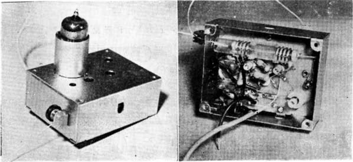
FM チューナ・ユニット, スター FU-30 形
