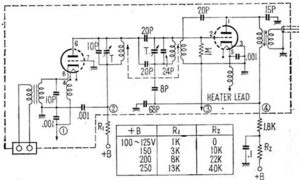
μ 同調 FM バック, スター FU-30 形の配線図
