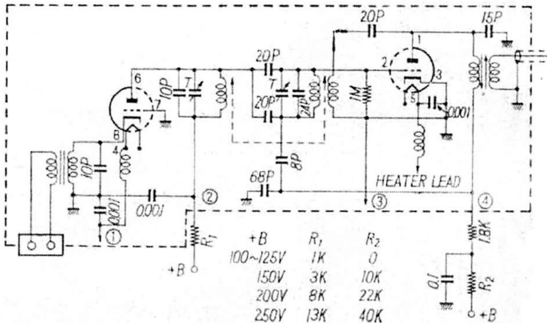
スターFU-35Bの回路図
