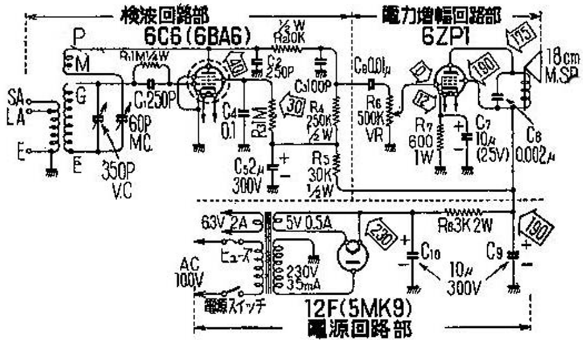
3球ラジオの記号配線図
