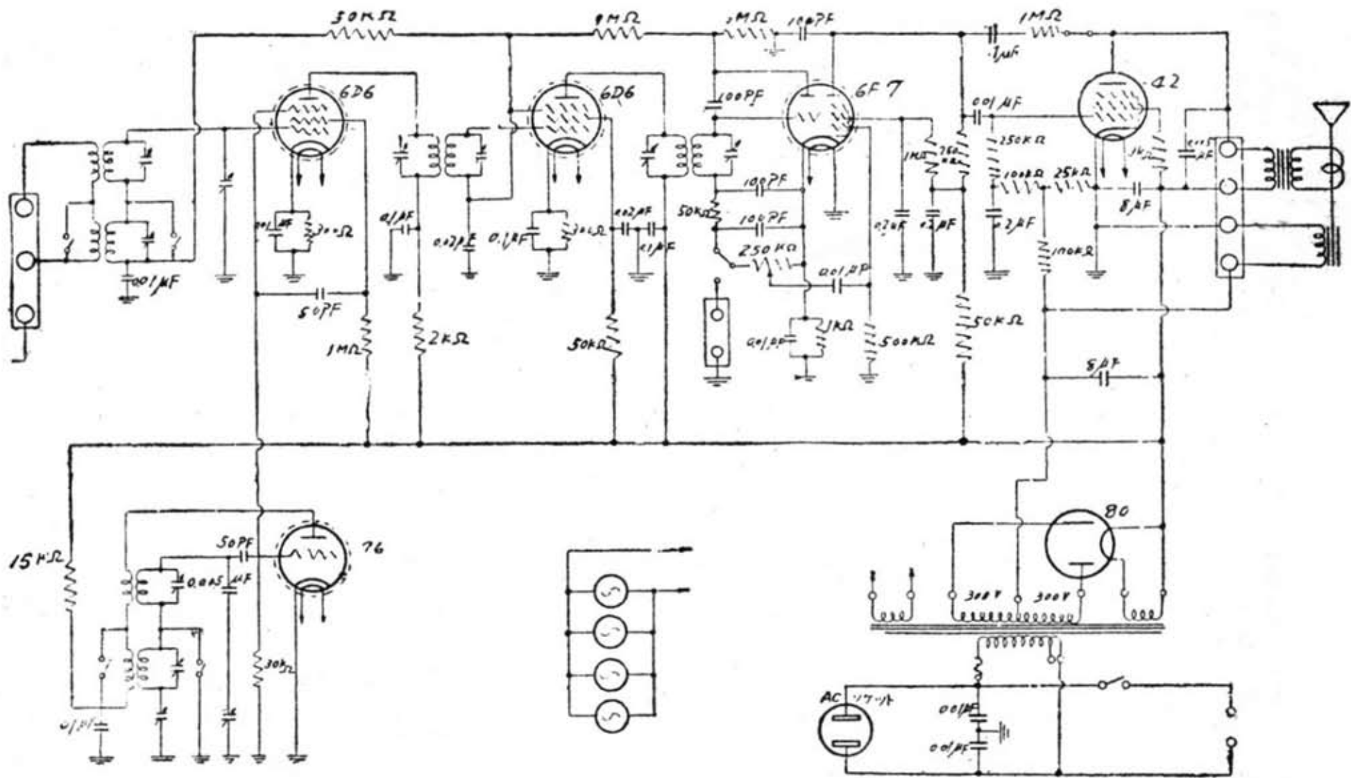
WORLD'S VOICE 配線圖
