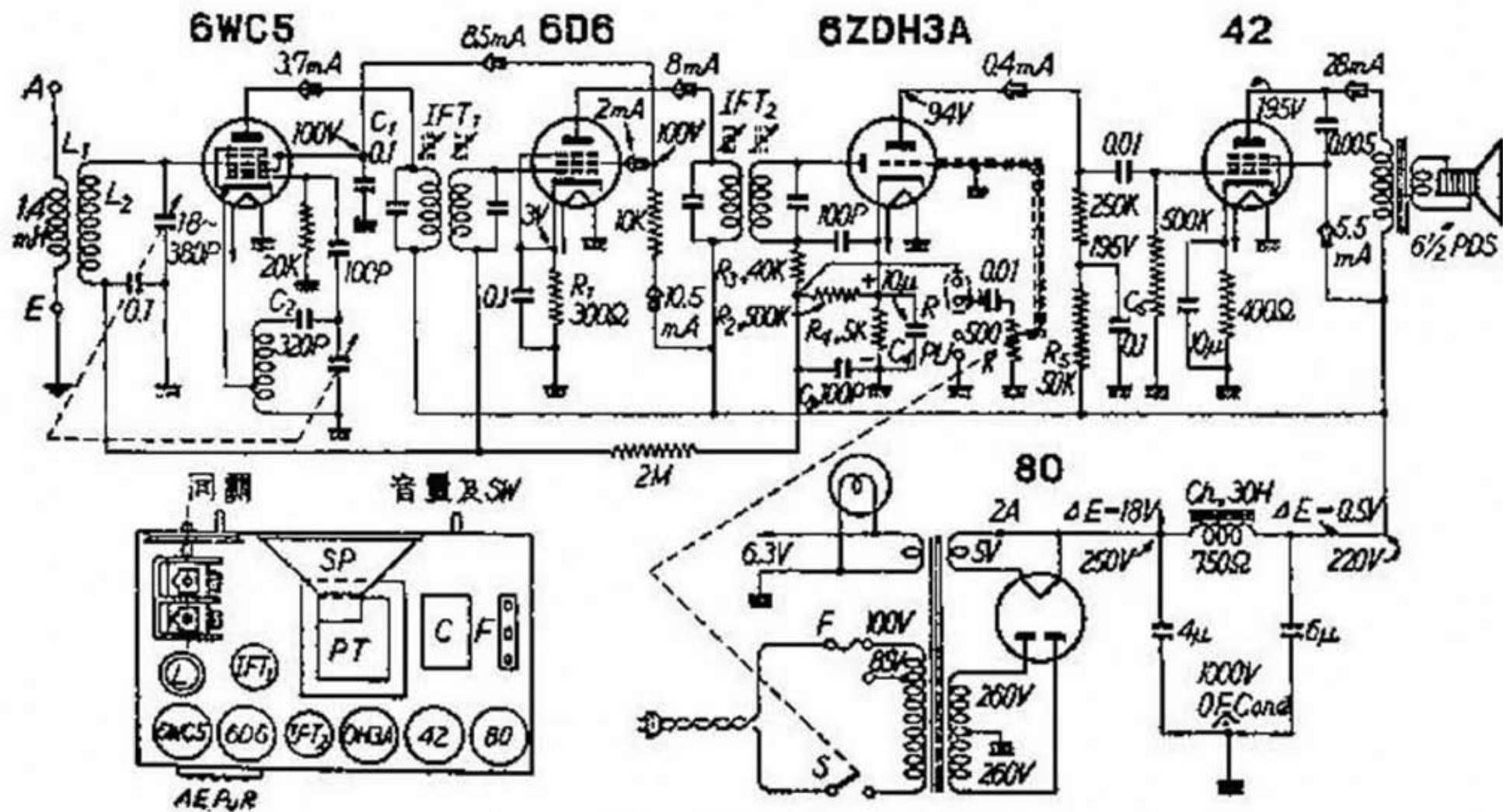
チン DR-1S5D 回路図
