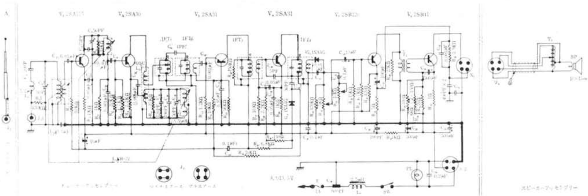
AR-68 配線図
