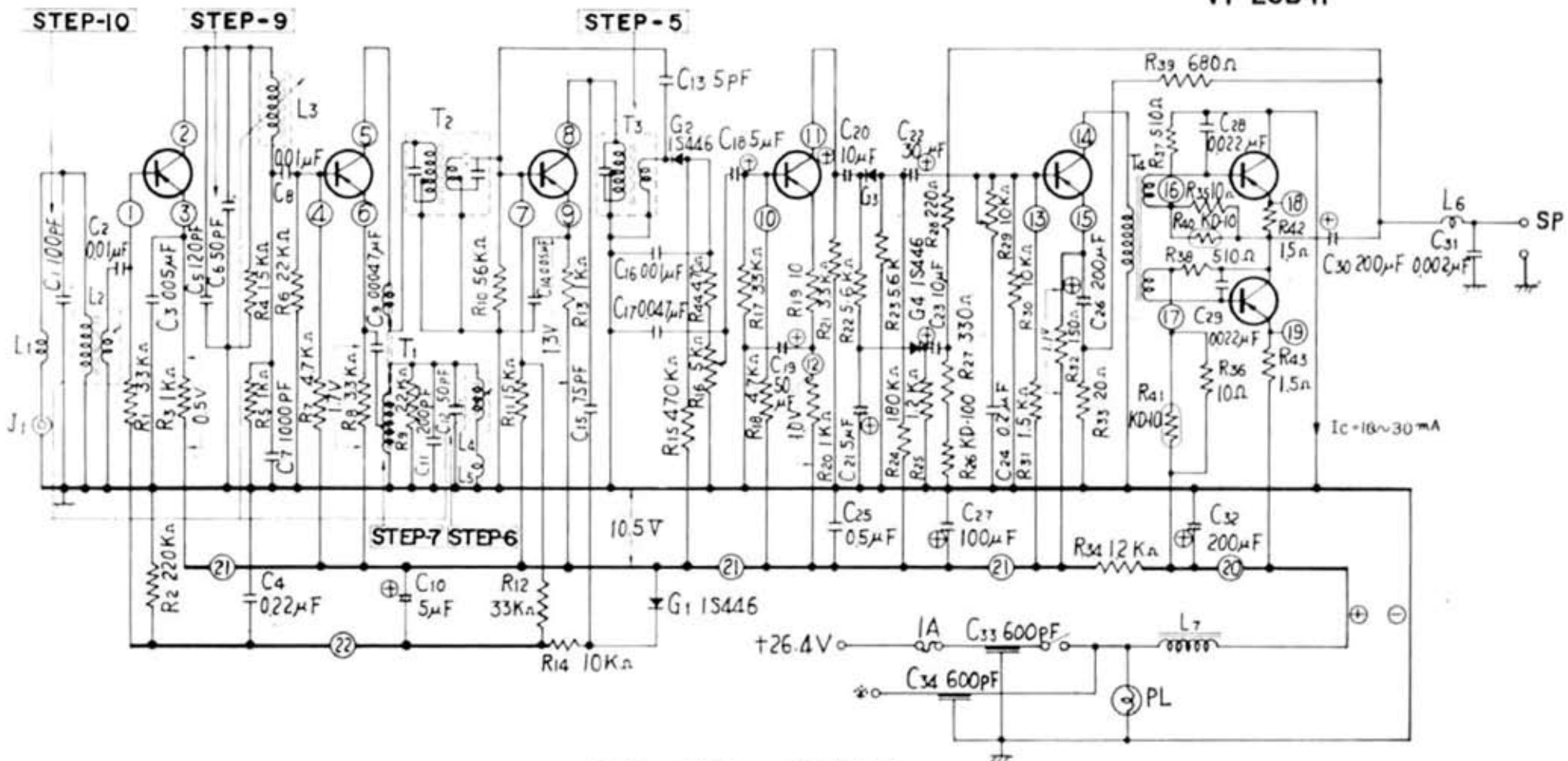
AT-1030 結線図
