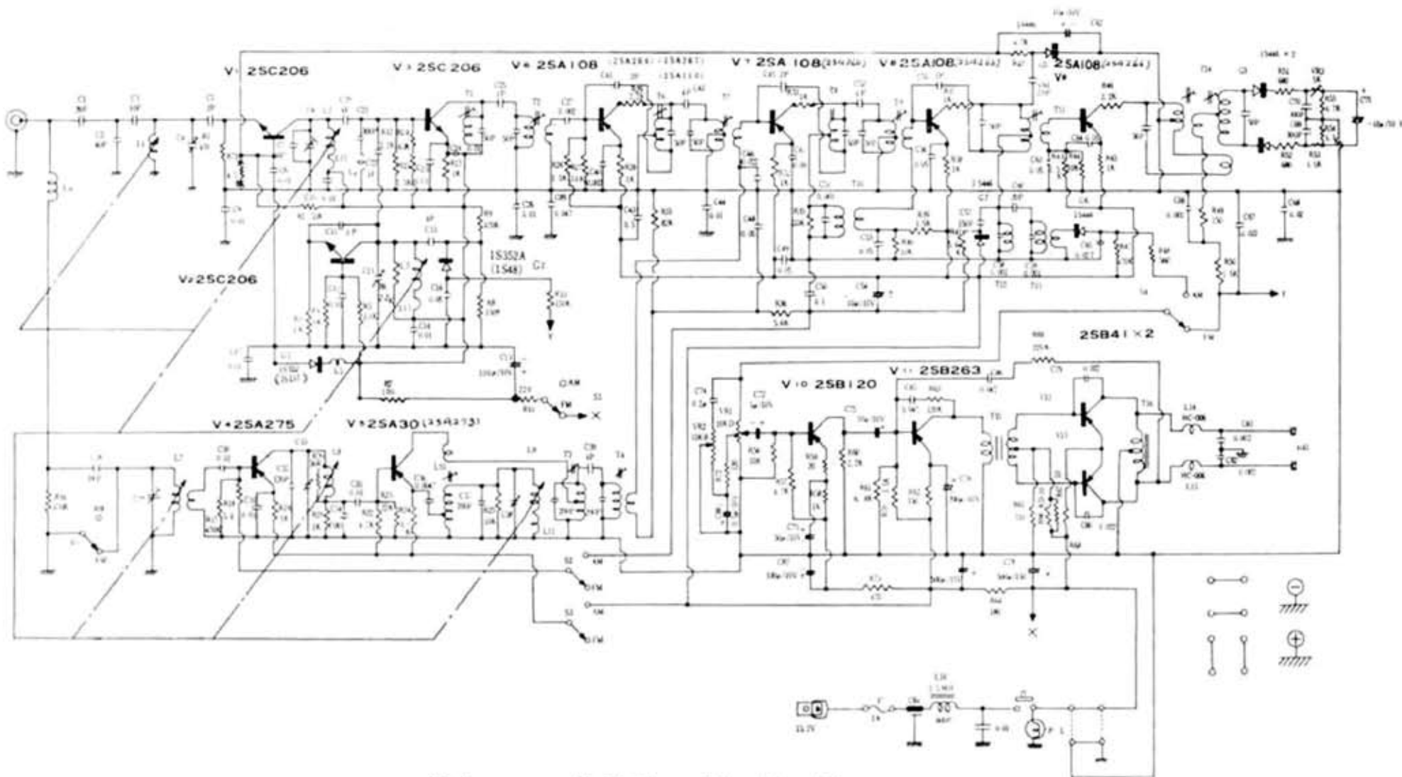
FA-205EX型 結線図
