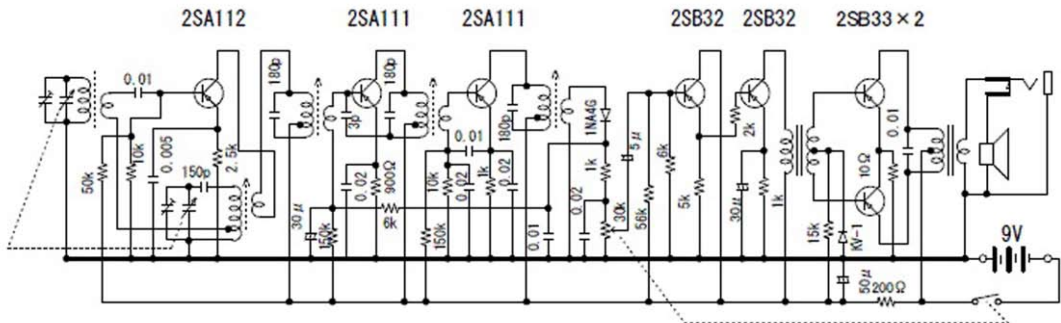
神戸工業 KT-75 回路図
